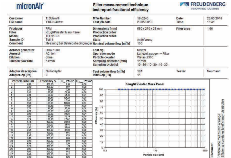
Partikelfilter Mars TFH91-03 Messung AC_fine bei 100m³/h Anlieferung
